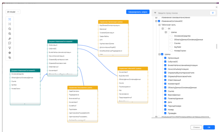
Рисунок. Детальная ER – модель отображения данных
